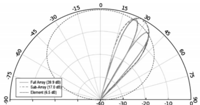
Formation of analog (sub-array) beams
